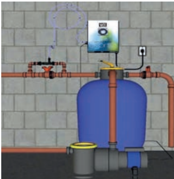
Diagrama de instalação do Gerador de Ozônio LTO
